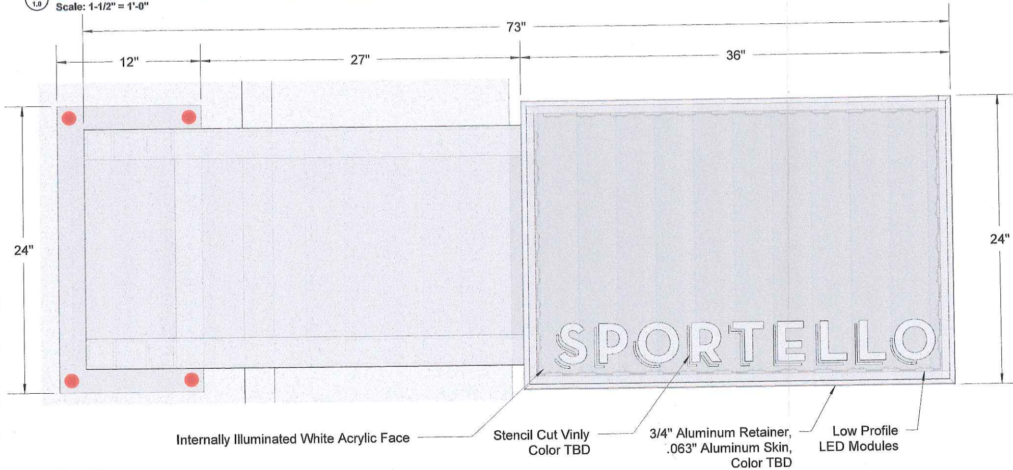
3 Front View Scale: 1-1/2" = 1'-0"
