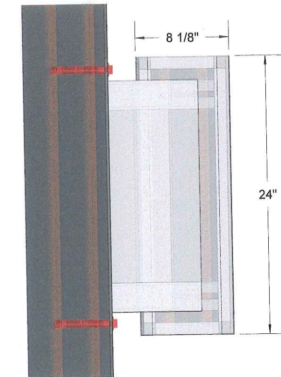
4 Left Side View Scale: 1-1/2" = 1'-0"
