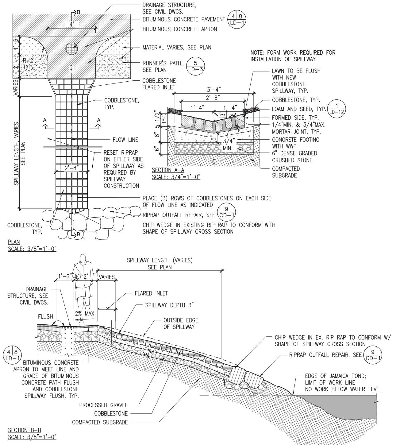
1 COBBLESTONE SPILLWAY SCALE: 3/8" = 1'-0"
