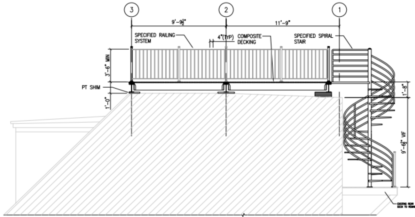
2 SECTION SCALE: 1/4" = 1'-0"
