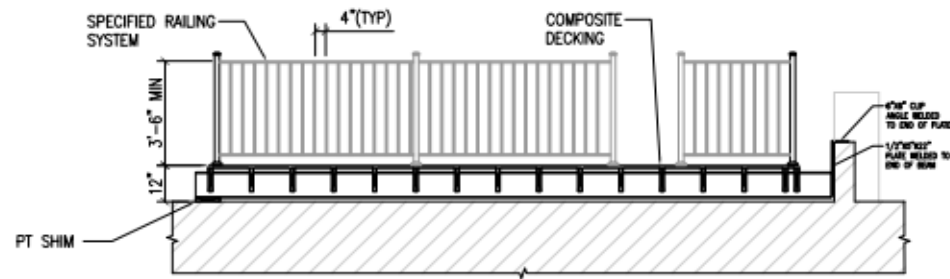
1 SECTION SCALE: 1/4" = 1'-0"
