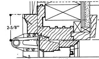
JAMB
